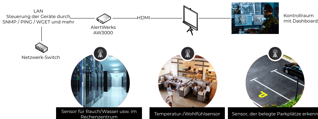
Verschiedene Sensoren für die Qualitätskontrolle
