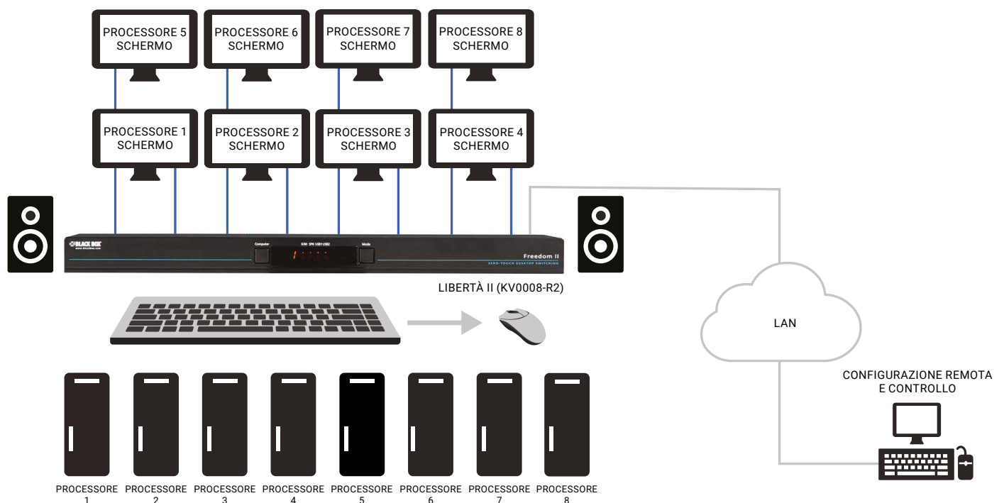
Configurazione a 8 porte Freedom II
