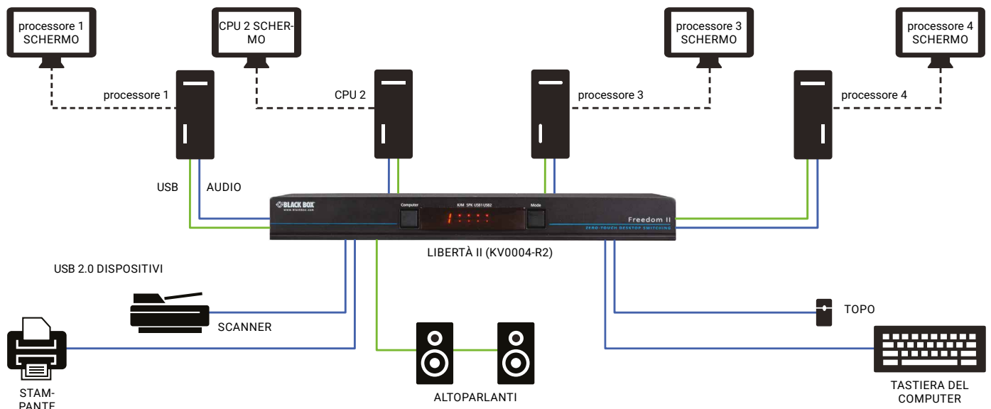
Configurazione Freedom II a 4 porte inclusi dispositivi USB 2.0
